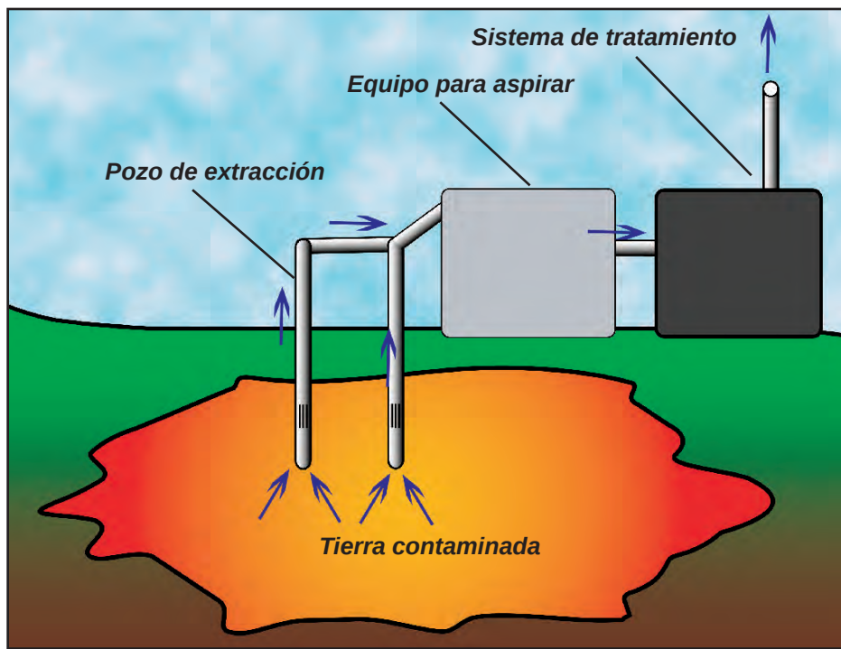
Un modelo del sistema de extracción de vapor en la tierra.
